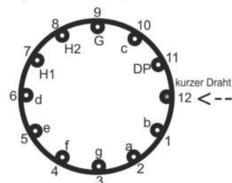
Ansicht von unten, IV-3A + IV-6
